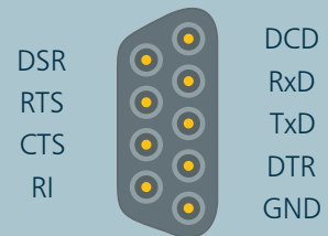
RS-232
